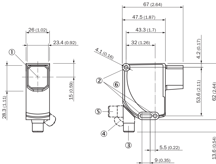
Rysunek wymiarowy Sensing distance from leading edge of lens
