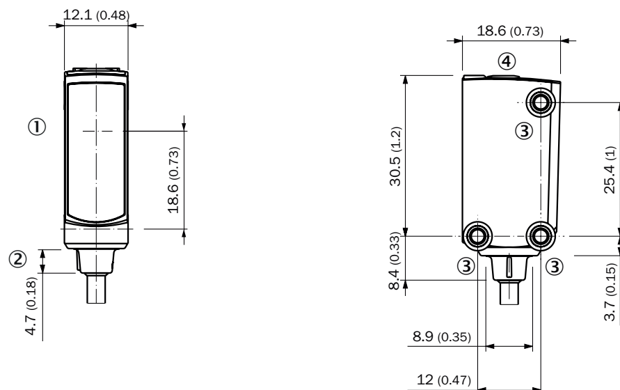
Rysunek wymiarowy, czujnik
