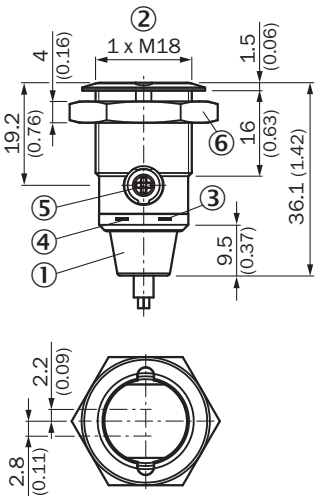
Rysunek wymiarowy GR18S, metal, przewód, osiowy, zalewalny (fully flush), możliwość ustawienia
