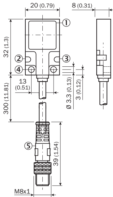
Rysunek wymiarowy IQ20, przewód z wtykiem M8, 3-pinowy
