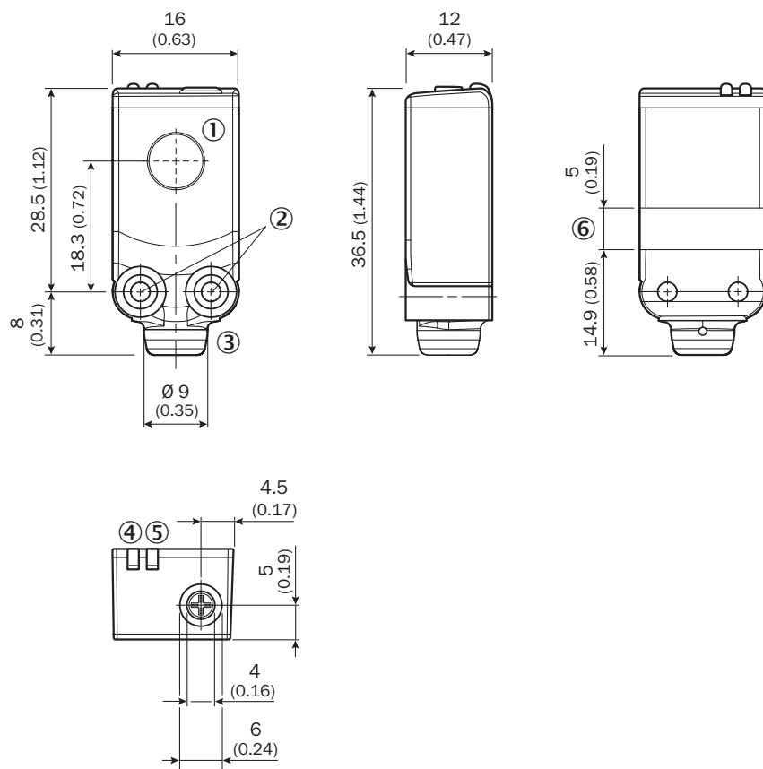
Rysunek wymiarowy CQ4, przewód z wtykiem
