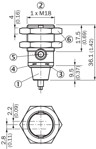
Rysunek wymiarowy GR18S, metal, przewód, osiowy
