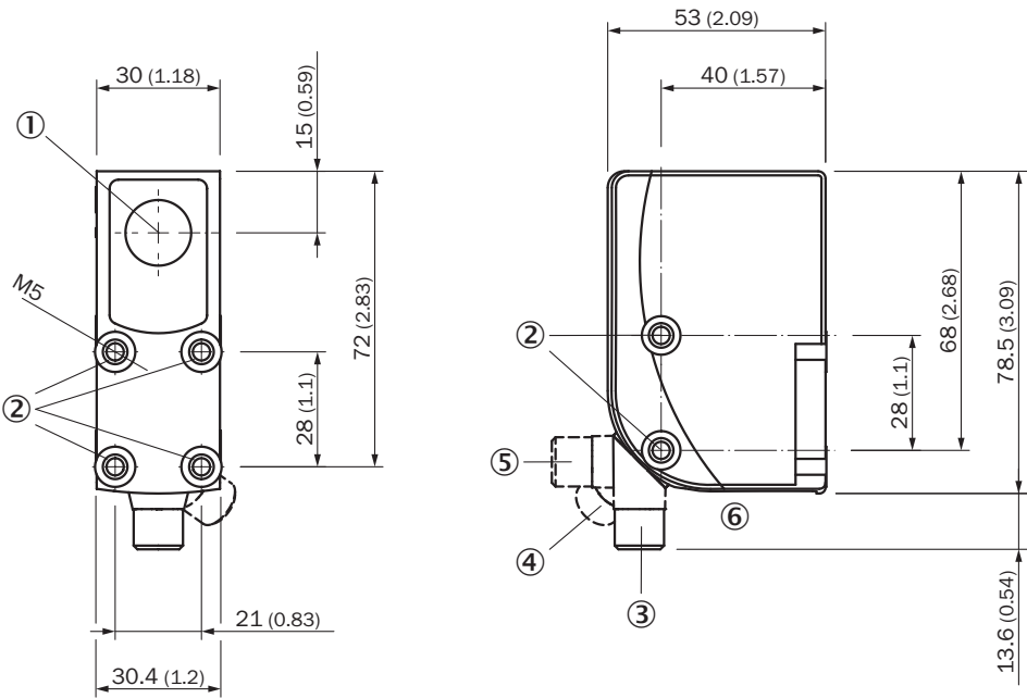
Wymiary w mm ① oś optyczna
