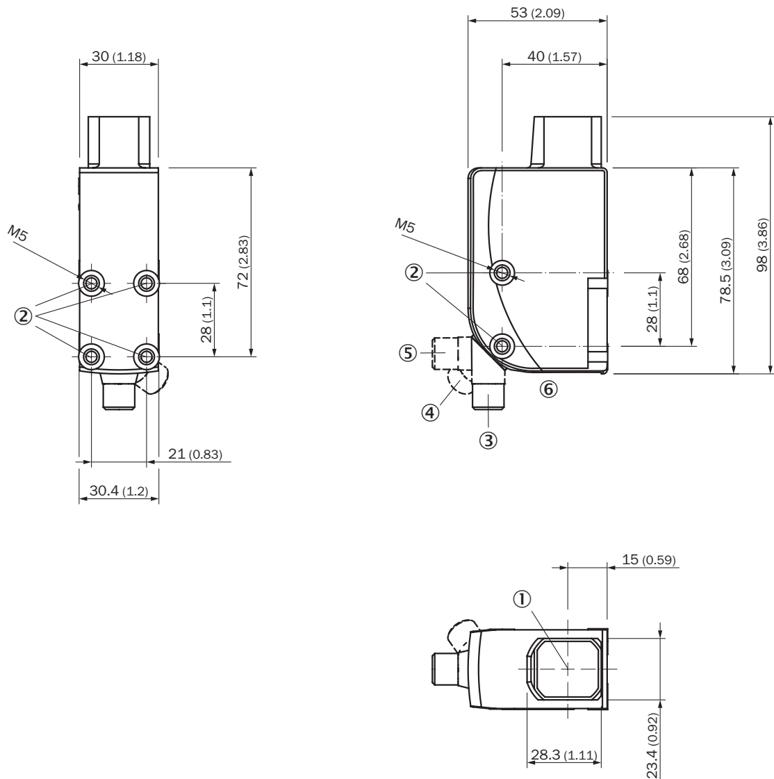
Rysunek wymiarowy Sensing distance from leading edge of lens
