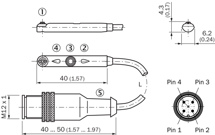
Rysunek wymiarowy Przewód z wtykiem M12, ze złączem radełkowym
