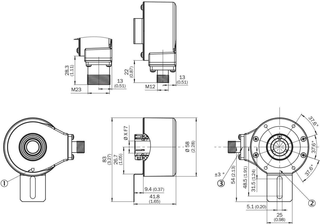
Rysunek wymiarowy
