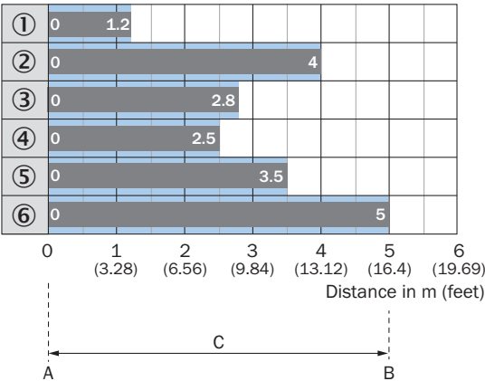
Wykres zasięgu wykrywania WLG16P-xxxxx1xx
