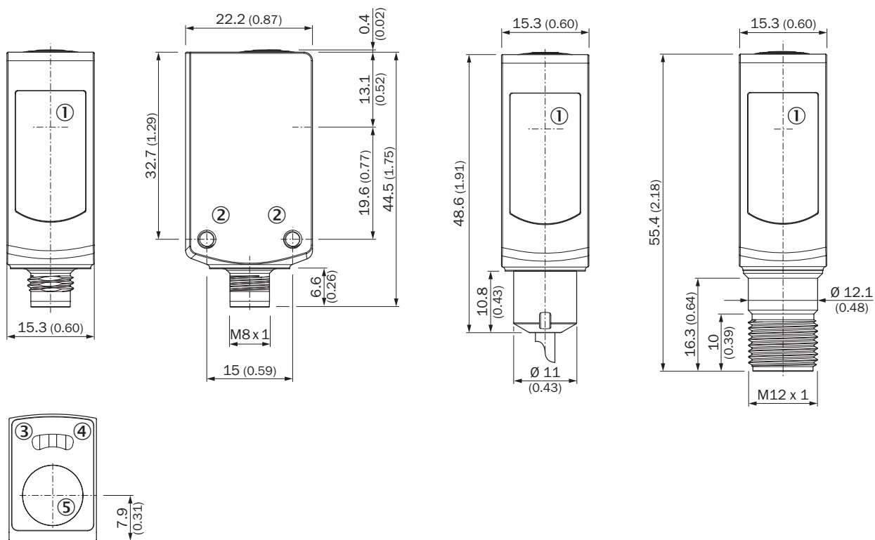
Rysunek wymiarowy WL4S-3V, WL4S-3V, z przyciskiem Teach-in
