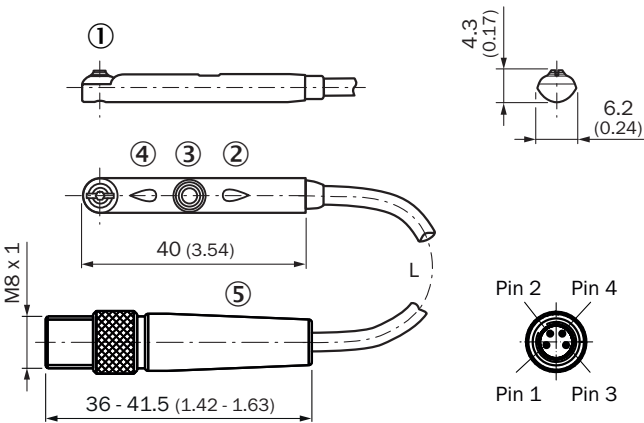
Rysunek wymiarowy Przewód z wtyczką M8, z radełkowanym złączem śrubowym
