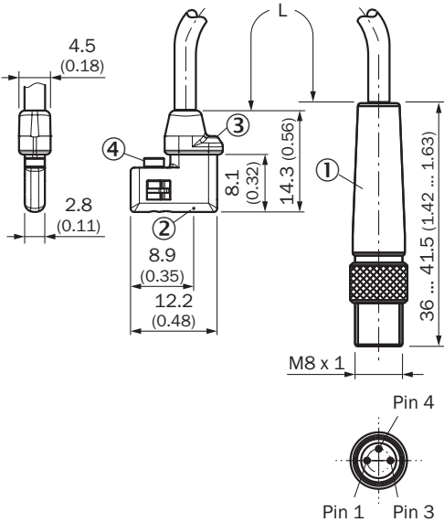
Rysunek wymiarowy Przewód z wtykiem, M8, ze złączem radełkowym
