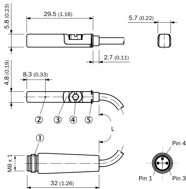
Rysunek wymiarowy Przewód z wtykiem M8
