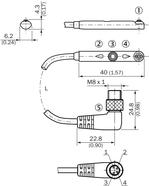
Rysunek wymiarowy Przewód z wtykiem M8, 4 piny, kątowny, ze złączem radełkowym
