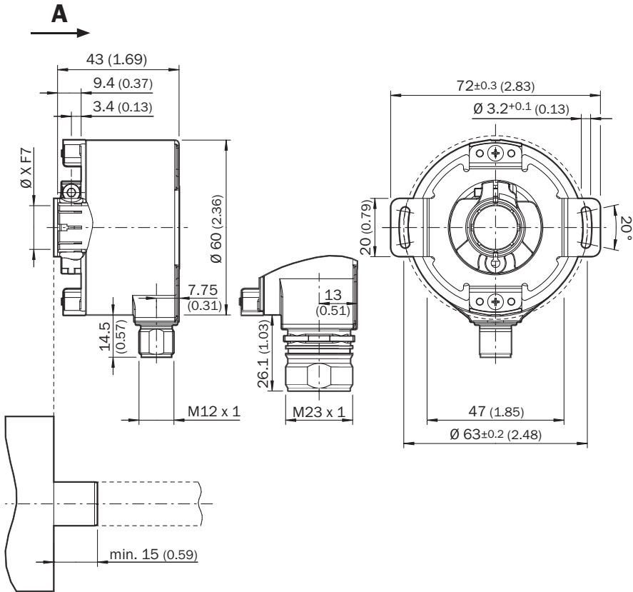
Rysunek wymiarowy
