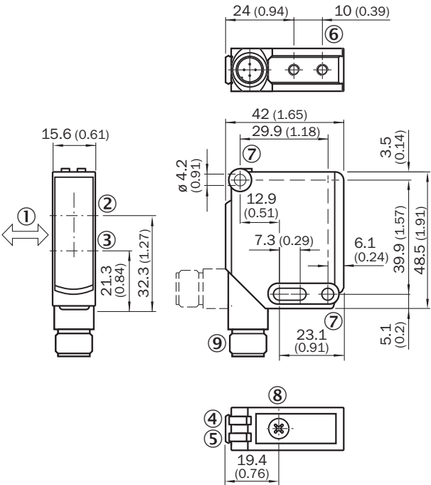
Rysunek wymiarowy WTB12-3, potencjometr
