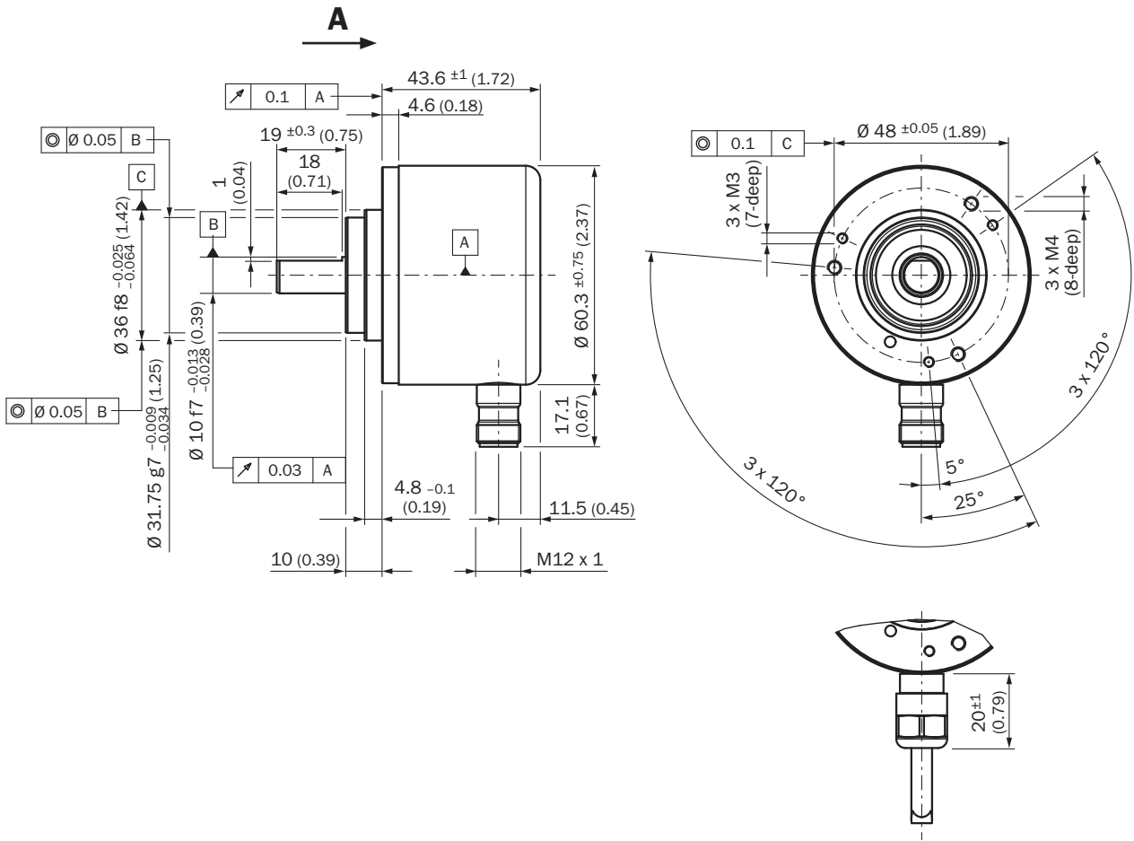
Rysunek wymiarowy
