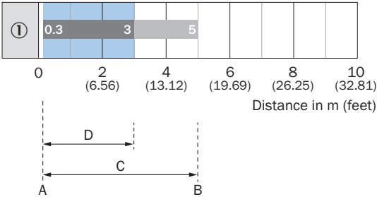
Wykres zasięgu wykrywania
