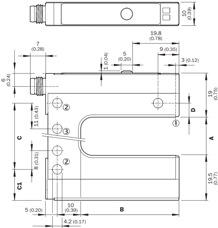
Rysunek wymiarowy Przycisk Teach-in WFL
