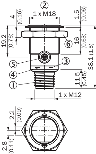
Rysunek wymiarowy GR18S, metal, wtyk, osiowy, zalewalny (fully flush), możliwość ustawienia
