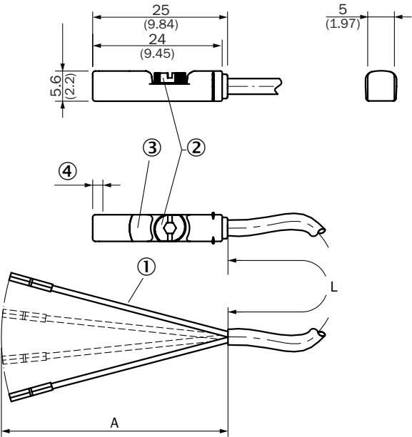
Rysunek wymiarowy Przewód
