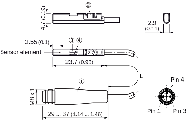
Rysunek wymiarowy Przewód z wtykiem M8
