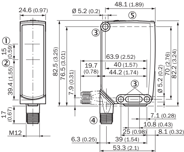
Rysunek wymiarowy, czujnik
