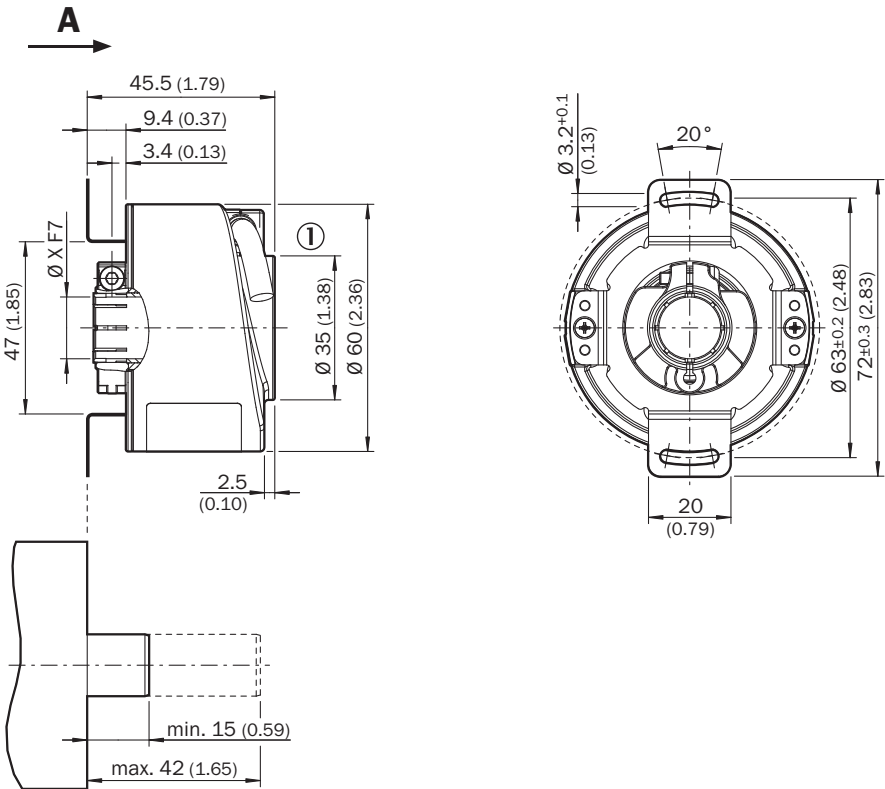
Wymiary w mm ① średnica przewodu = 5,6 mm +/- 0,2 mm, promień gięcia = 30 mm
