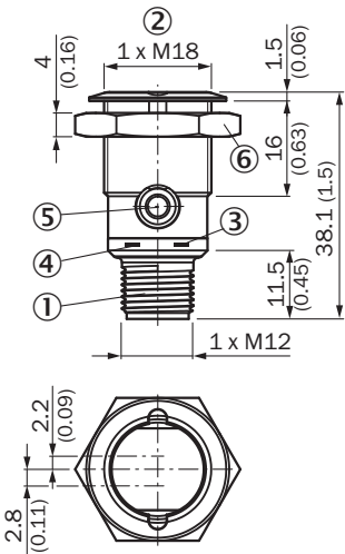
Rysunek wymiarowy GR18S, metal, wtyk, osiowy, zalewalny (fully flush)
