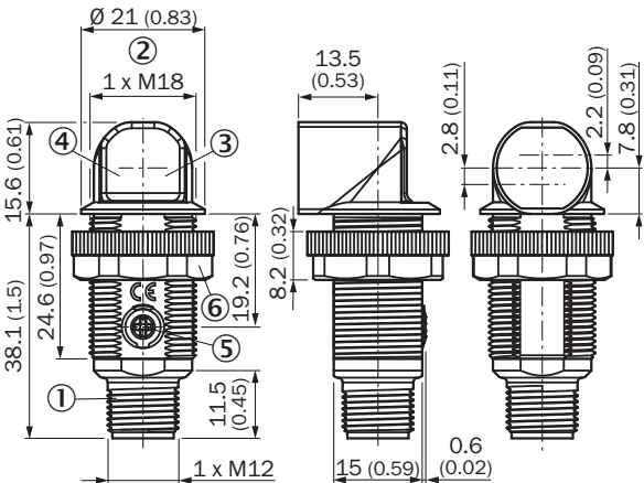
Rysunek wymiarowy GR18S, tworzywo sztuczne, wtyk, kątowy
