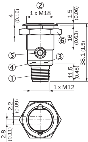
Rysunek wymiarowy GR18S, metal, wtyk, osiowy, zalewalny (fully flush)
