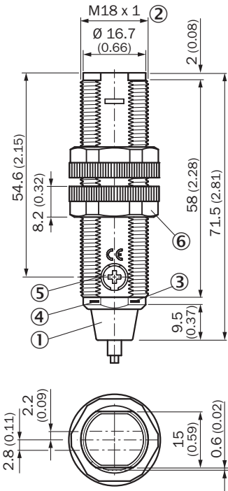
Rysunek wymiarowy GRTE18, GRL18, GRSE18, tworzywo sztuczne, przewód, osiowy
