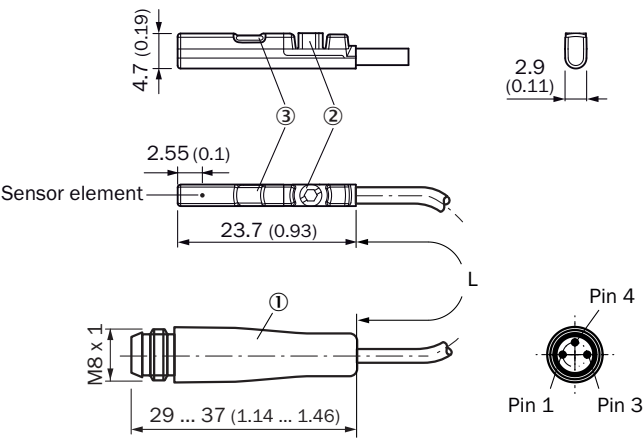
Rysunek wymiarowy Przewód z wtykiem M8
