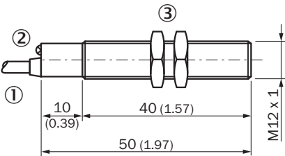
Rysunek wymiarowy MM12, przewód, standardowy
