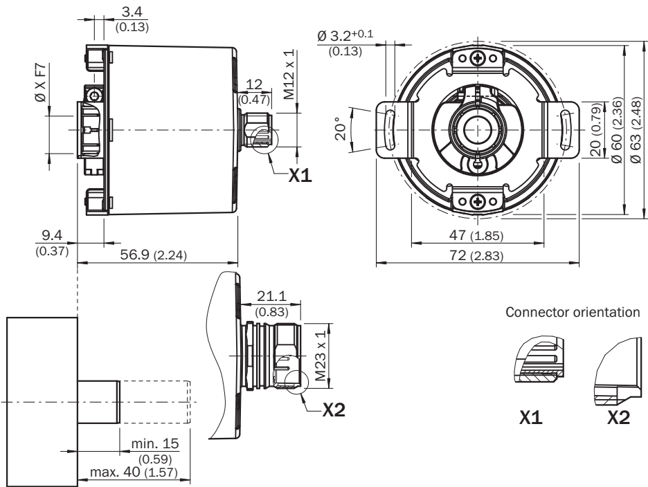
Rysunek wymiarowy Wersja z otworem nieprzelotowym, wtyk osiowy M12 i M23
