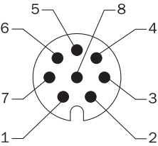
widok wtyczki urządzenia M12 na przewodzie/obudowie
