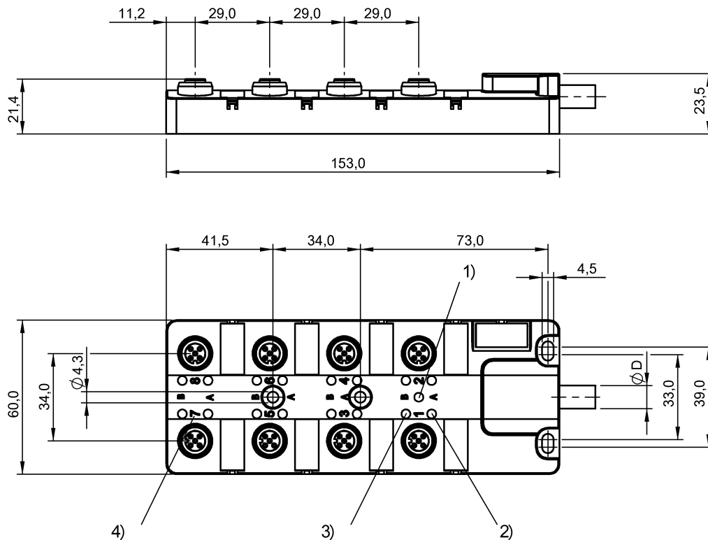
1) Wskaźnik uruchomienia, zielony 2) Dioda LED żółta dla sygnału 1 (NO) 3) Dioda LED żółta dla sygnału 2 (NC) 4) Numeracja miejsc wtykowych
