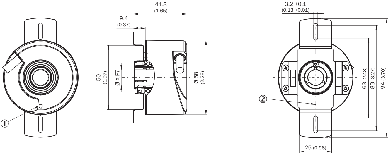
Rysunek wymiarowy
