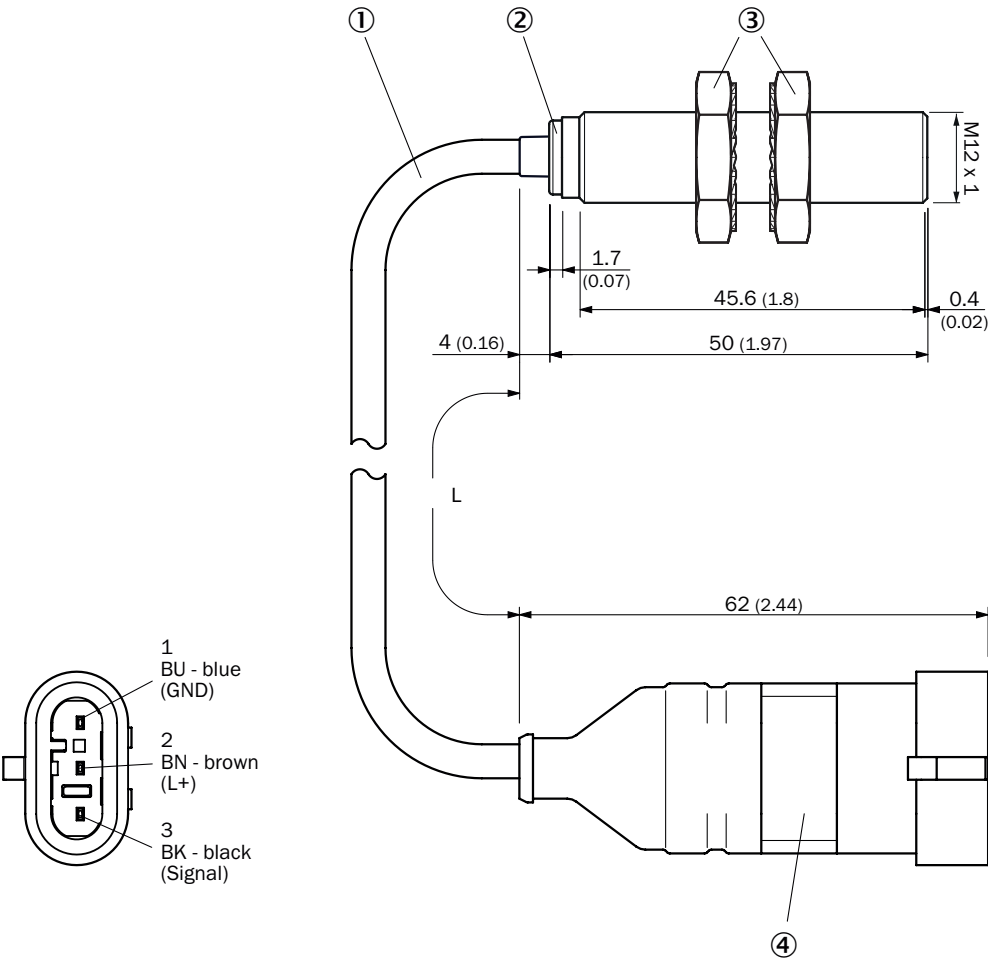
Rysunek wymiarowy Konstrukcja standardowa IMB12, przewód z wtykiem AMP, zabudowany
