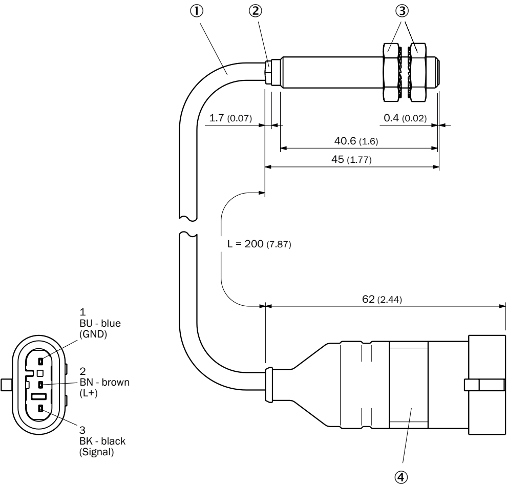
Rysunek wymiarowy Konstrukcja standardowa IMB08, przewód z wtykiem AMP, zabudowany
