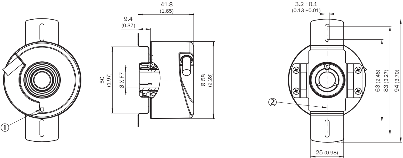
Rysunek wymiarowy
