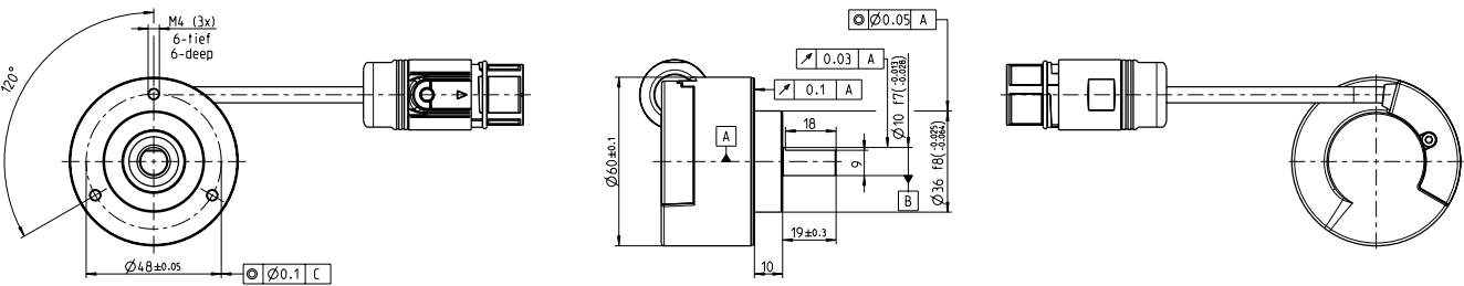
Wymiary w mm
