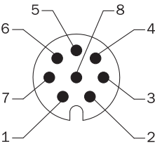
widok wtyczki urządzenia M12 na przewodzie/obudowie
