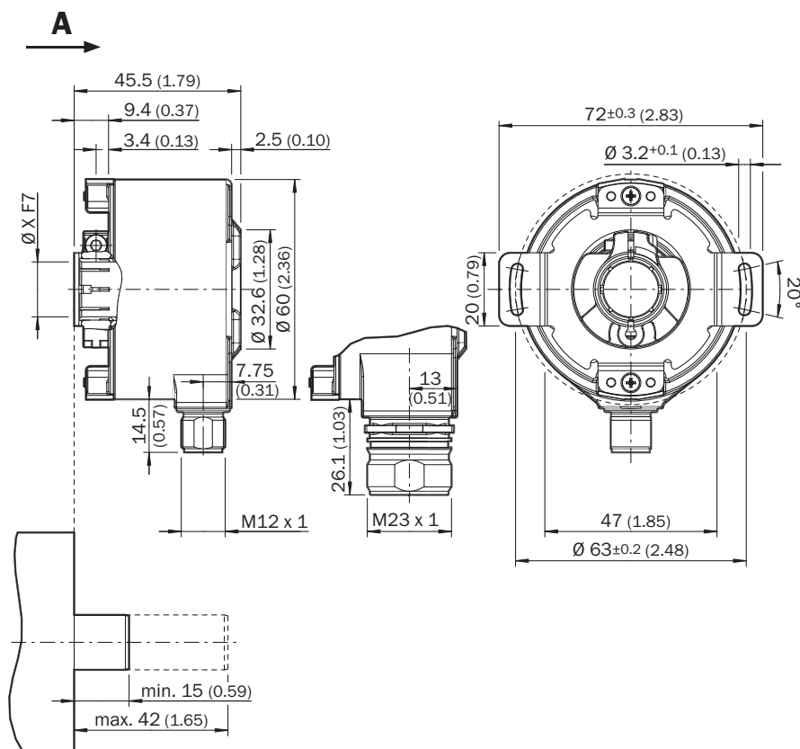
Rysunek wymiarowy Otwór nieprzelotowy, wtyk promieniowy M12 i M23
