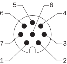
widok wtyczki urządzenia M12 na enkoderze
