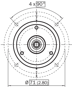
All dimensions in mm (inch) Numer artykułu 2029165
