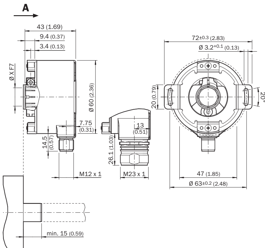
Rysunek wymiarowy (Wymiary w mm)
