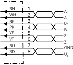
Przyporządkowanie styków
