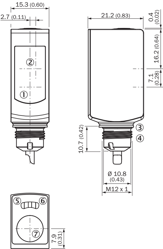
Rysunek wymiarowy Adapter z gwintem M12
