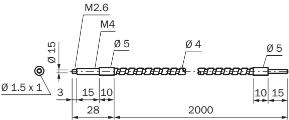
Rysunek wymiarowy LL3-TW01-2
