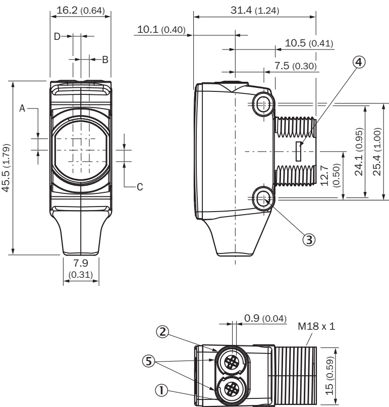
Rysunek wymiarowy
