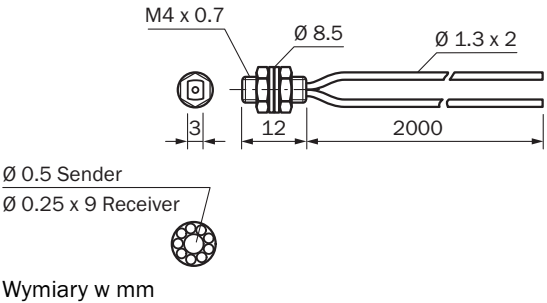
Rysunek wymiarowy LL3-DM02
